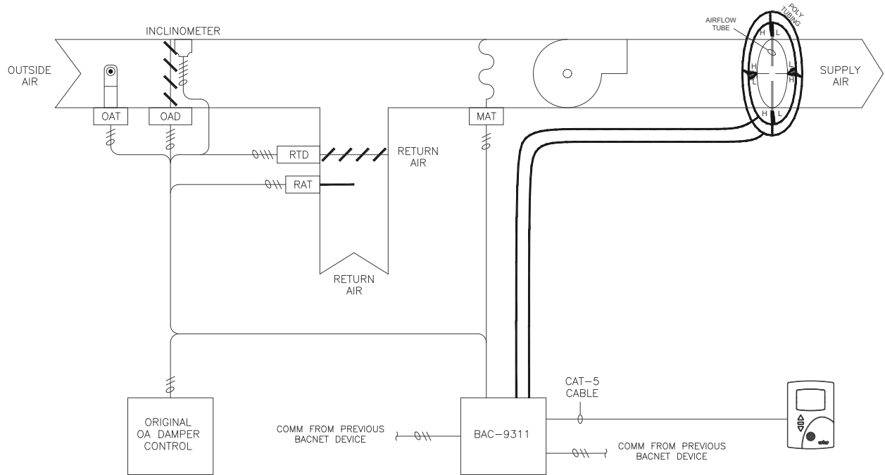
AFMS LAYOUT
