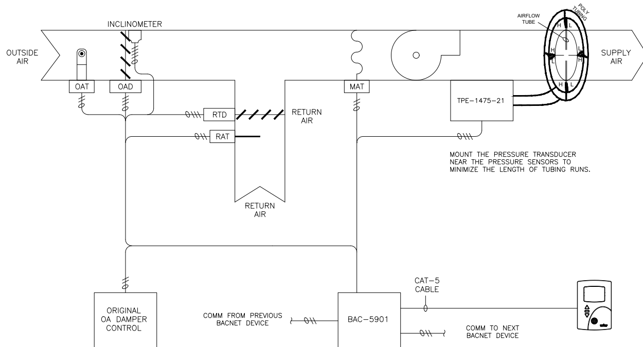
AFMS LAYOUT
