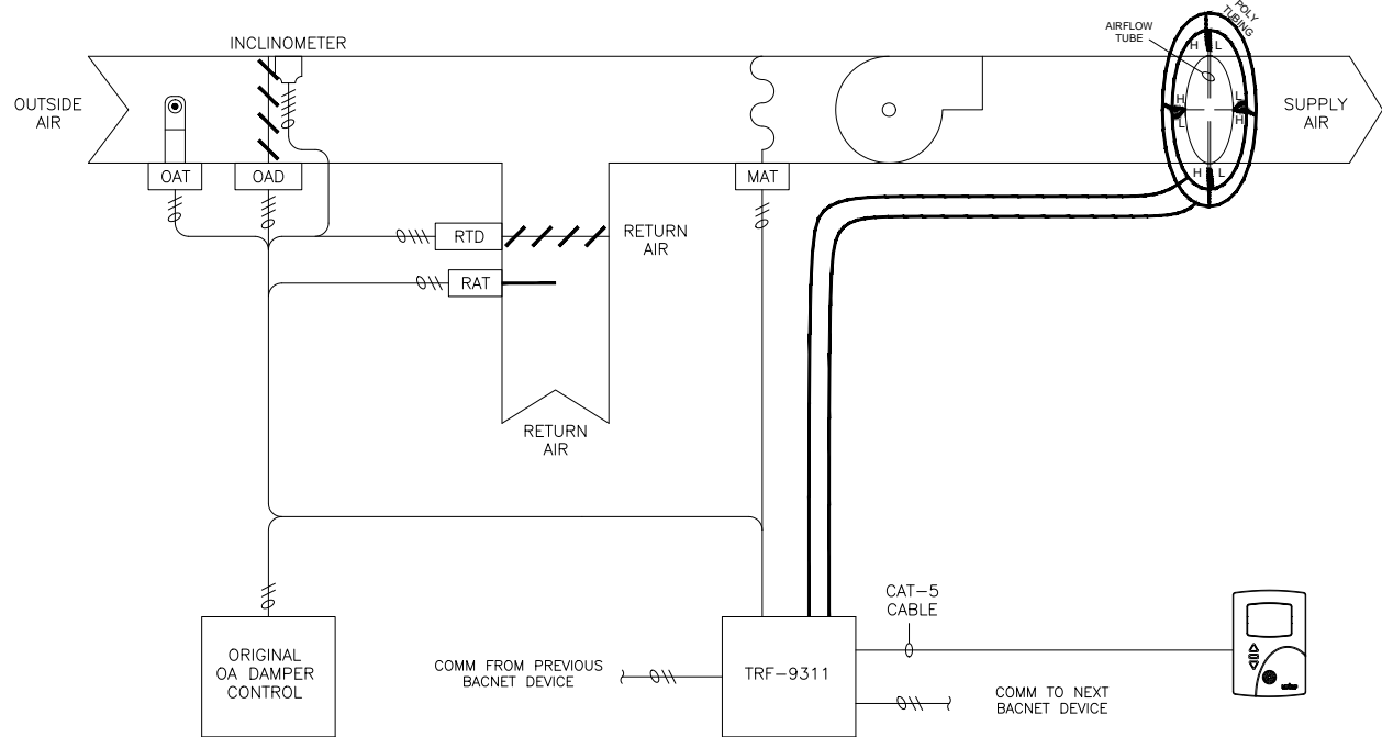
AFMS LAYOUT
